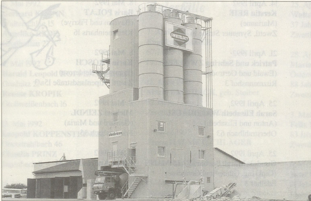
Das neue Swietelsky-Betonwerk, an das die Recyclinganlage direkt angeschlossen ist
